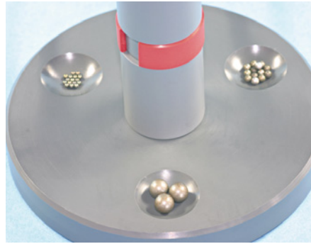
Messtativ mit Aussparungen zum sicheren Aufbewahren der Referenzkugeln während der Messung
