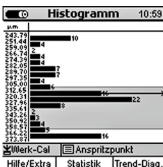
Histogramm und Trend-Diagramm mit MiniTest 7400 FH
